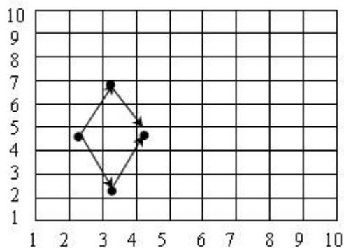
图 13-4 骑士游历
