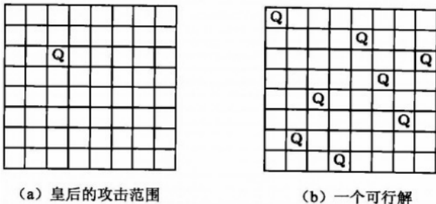
图 10-1 八皇后问题
