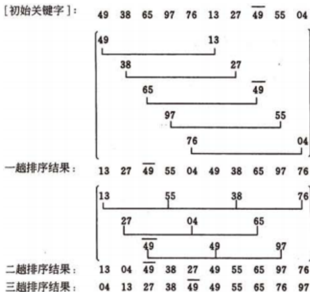
图 7-1 希尔排序
